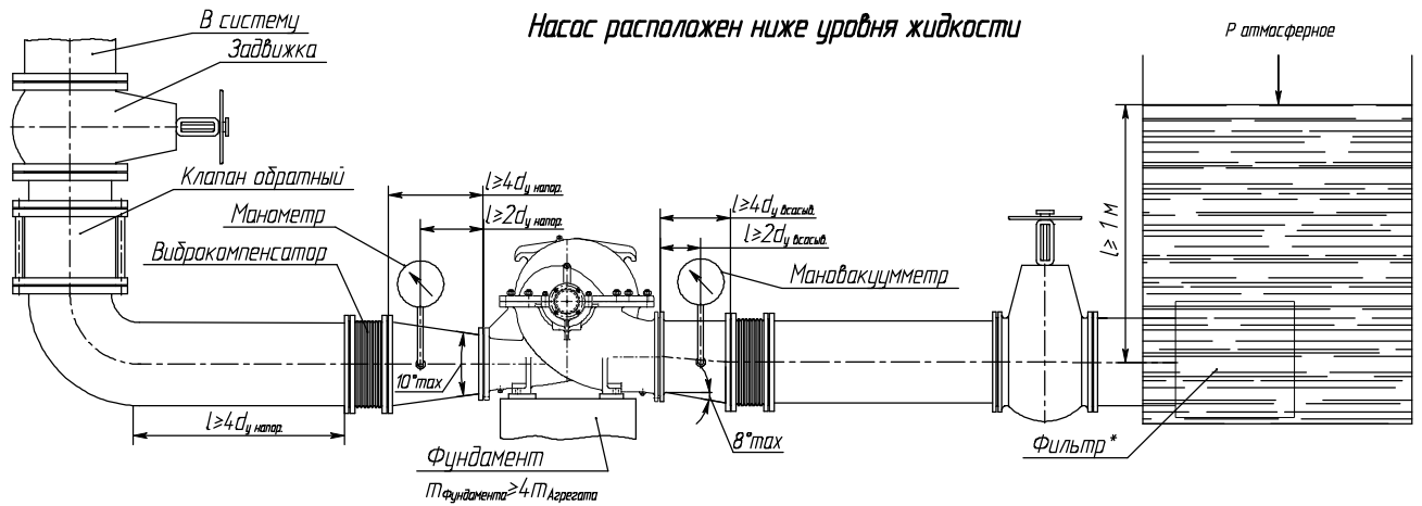
Схема - 2
