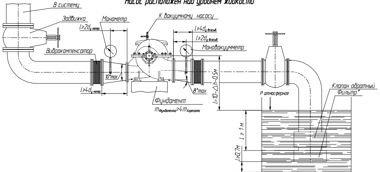
Схема – 1
