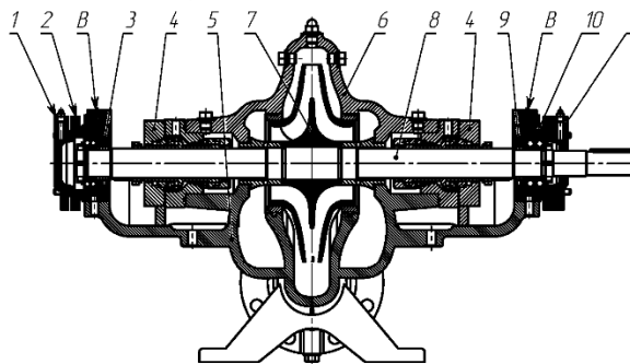
Насос центробежный типов ЦН160/112 и ЦН90/100
